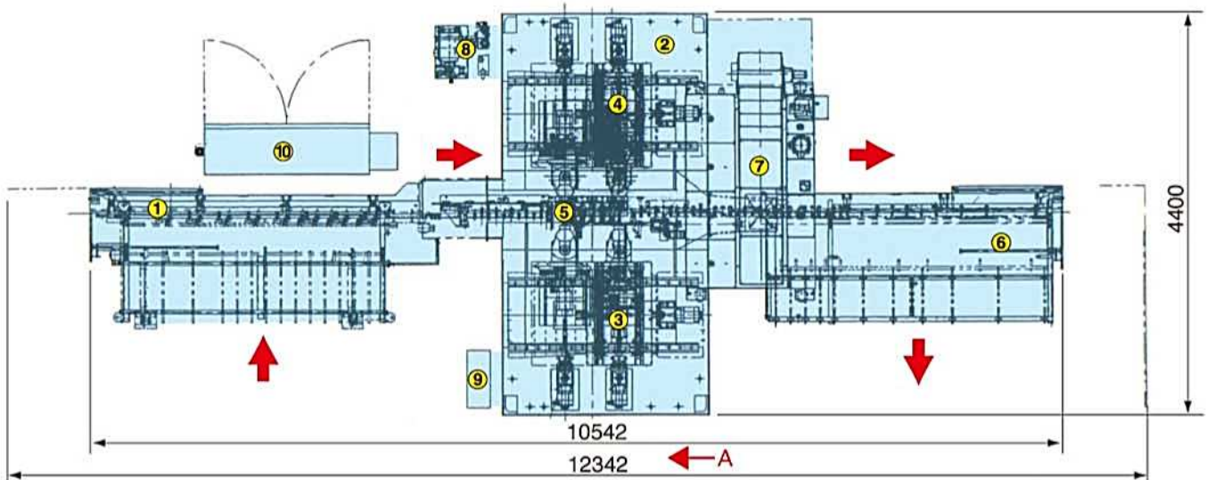
機械全体—搬入側
