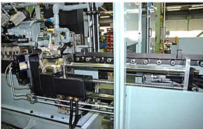
加工物位置決めピン、搬出装置—NC駆動（V軸）
