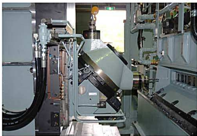
左側ターレットヘッド-2位置インデックス
