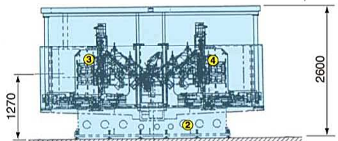
A視図
