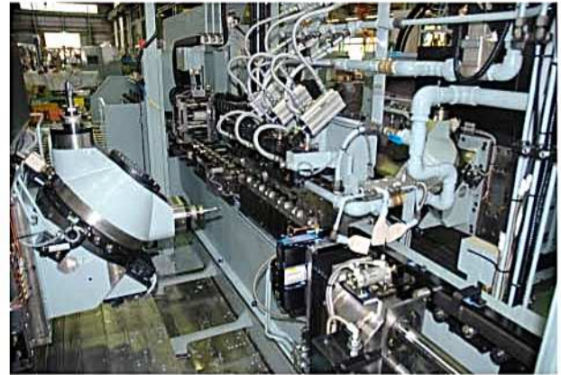
機械作業部
