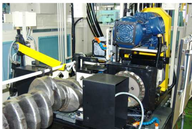
右側ヘッド部 手前側 ミーリングヘッドユニット 11kw、150rpm 奥側 センタードリルヘッドユニット 2.2kw、310rpm
