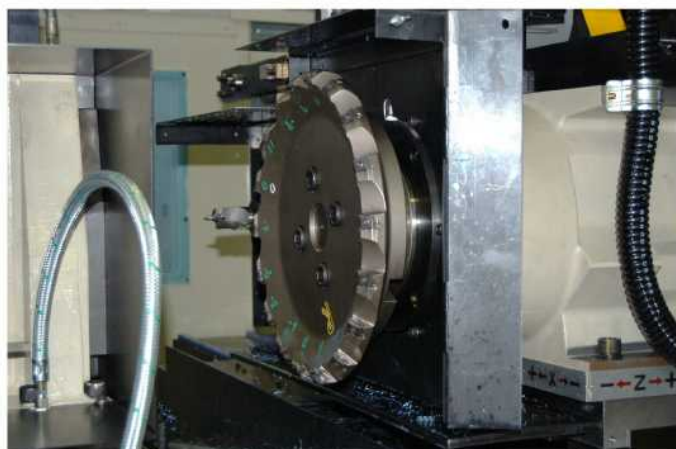
右側カッター及びドリル
