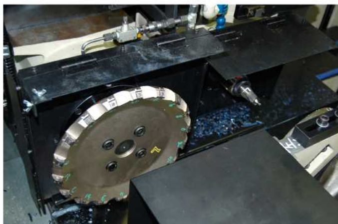
左側カッター及びドリル
