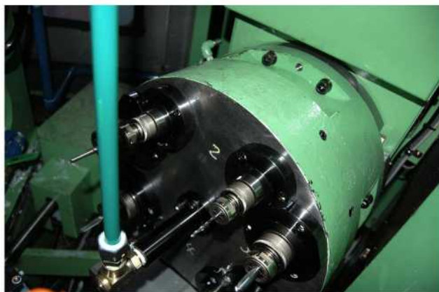
5STインレット穴、タップ穴
