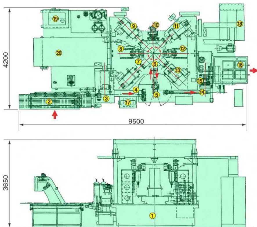
機械レイアウト
