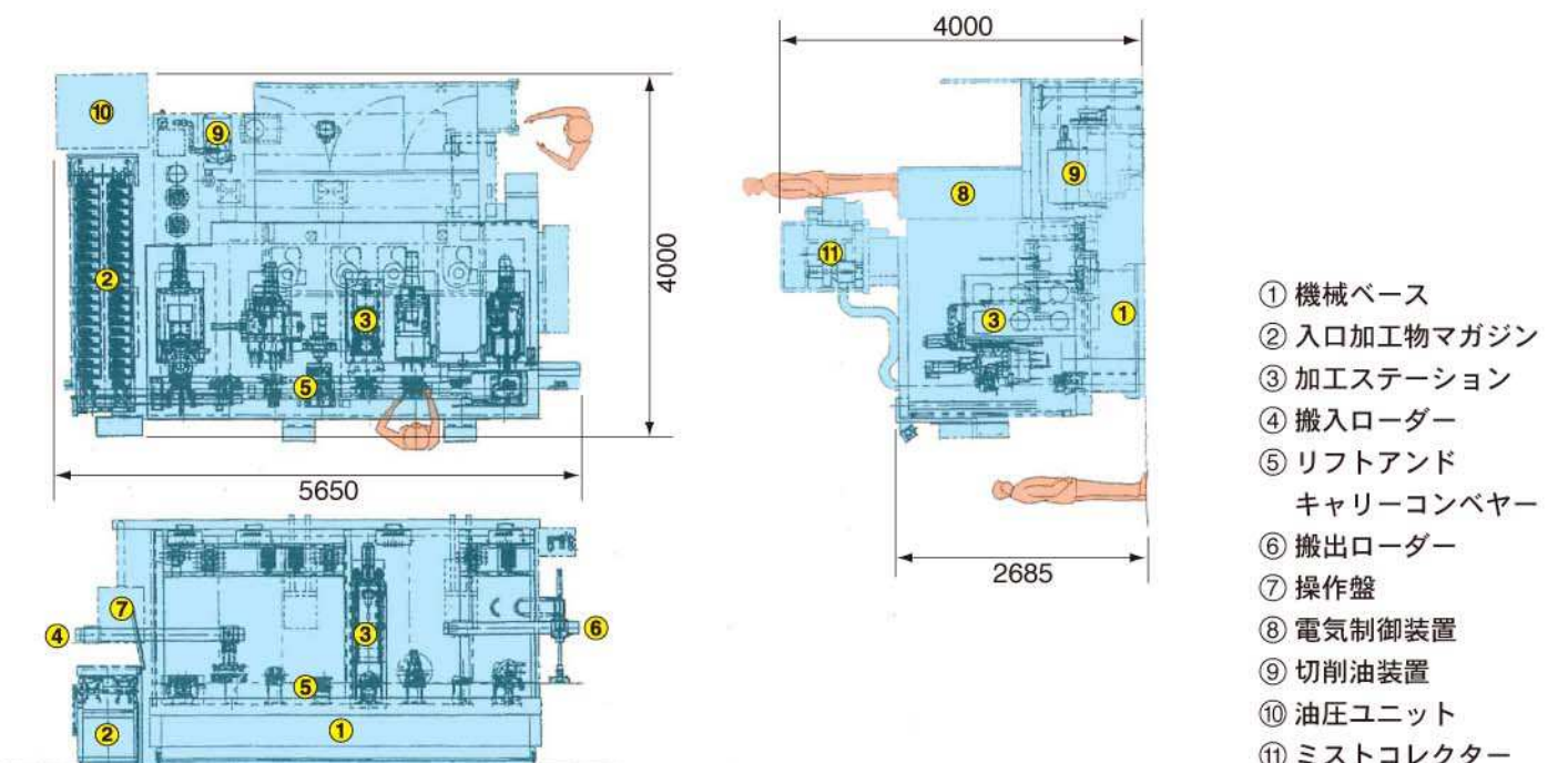
機械全体
