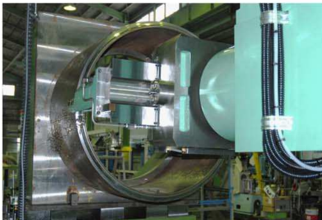
加工状況—機械側より見る
