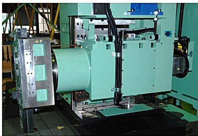
フェーシングヘッド 主軸径Φ200mm
