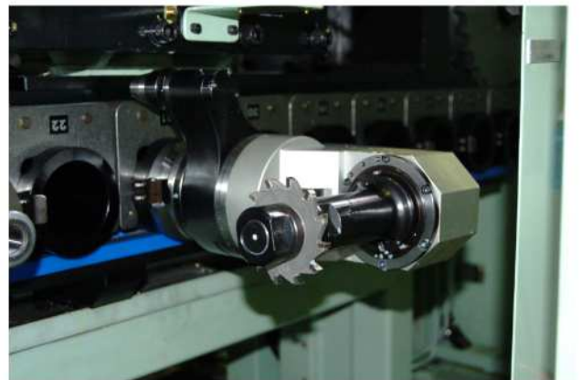
R面 切欠加工用工具
