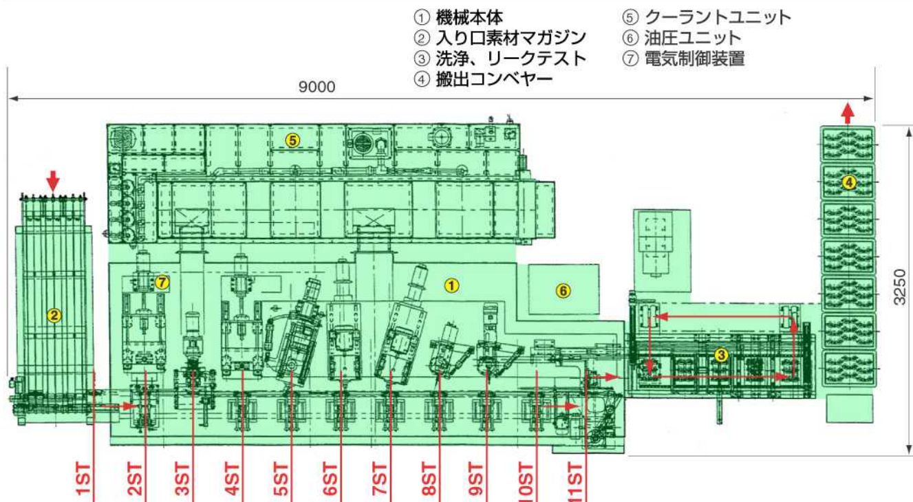
機械レイアウト (平面図)
