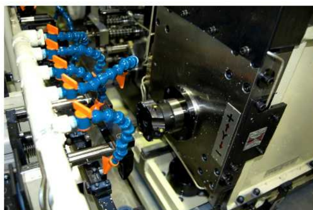
5ST回転機能付きMiヘッド
