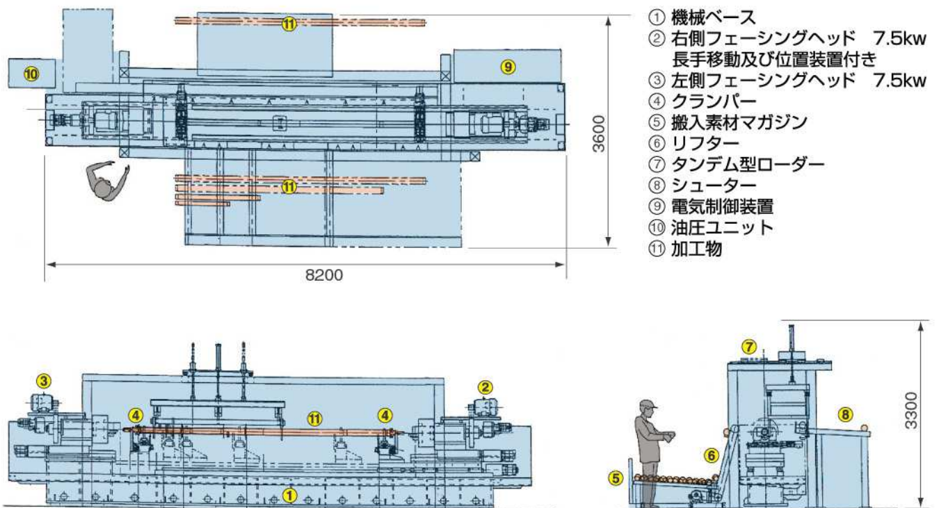
機械レイアウト図
