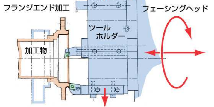
フェーシングヘッド部
