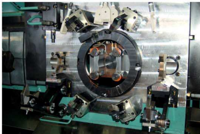
治具部、リング内側は加工物 センターリング装置
