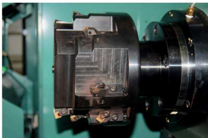
センター用ボーリング工具 3種類の加工物に対応します
