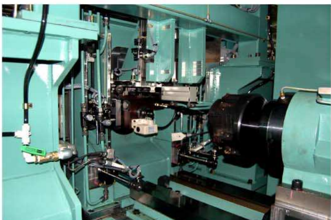
治具部裏側、加工物センターリング装置
