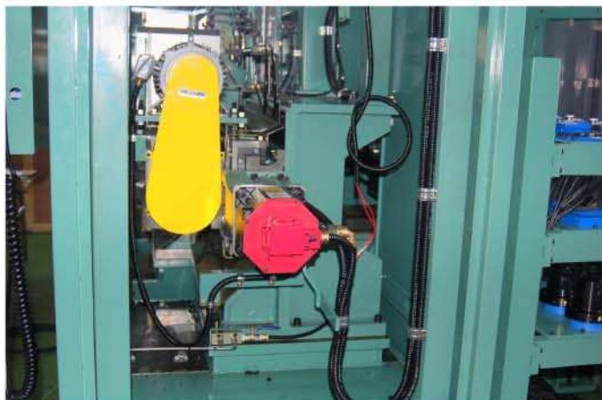
Rボーリングヘッド
